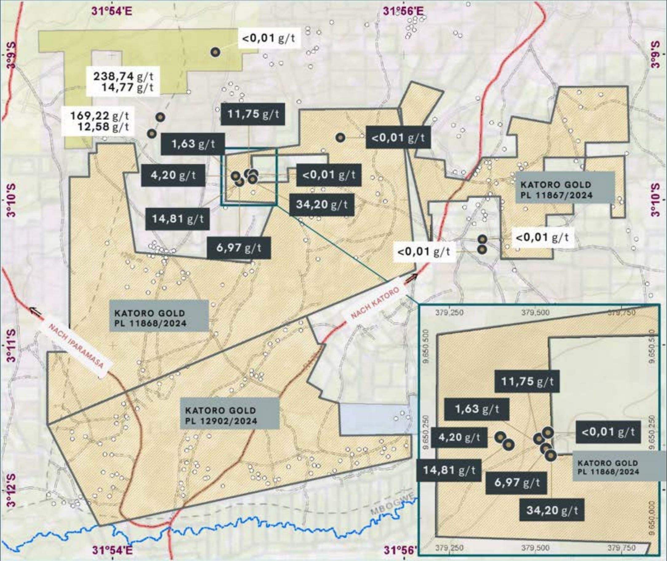
DIE KARTE ZEIGT DIE LAGE DER AUF UND RUND UM DIE GOLD-LIEGENSCHAFT KATORO ENTNOMMENEN PROBEN MIT GEHALTEN IN G/T AU.
